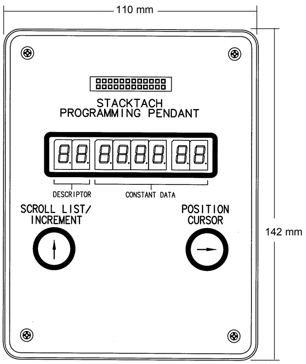
Programming Pendant
